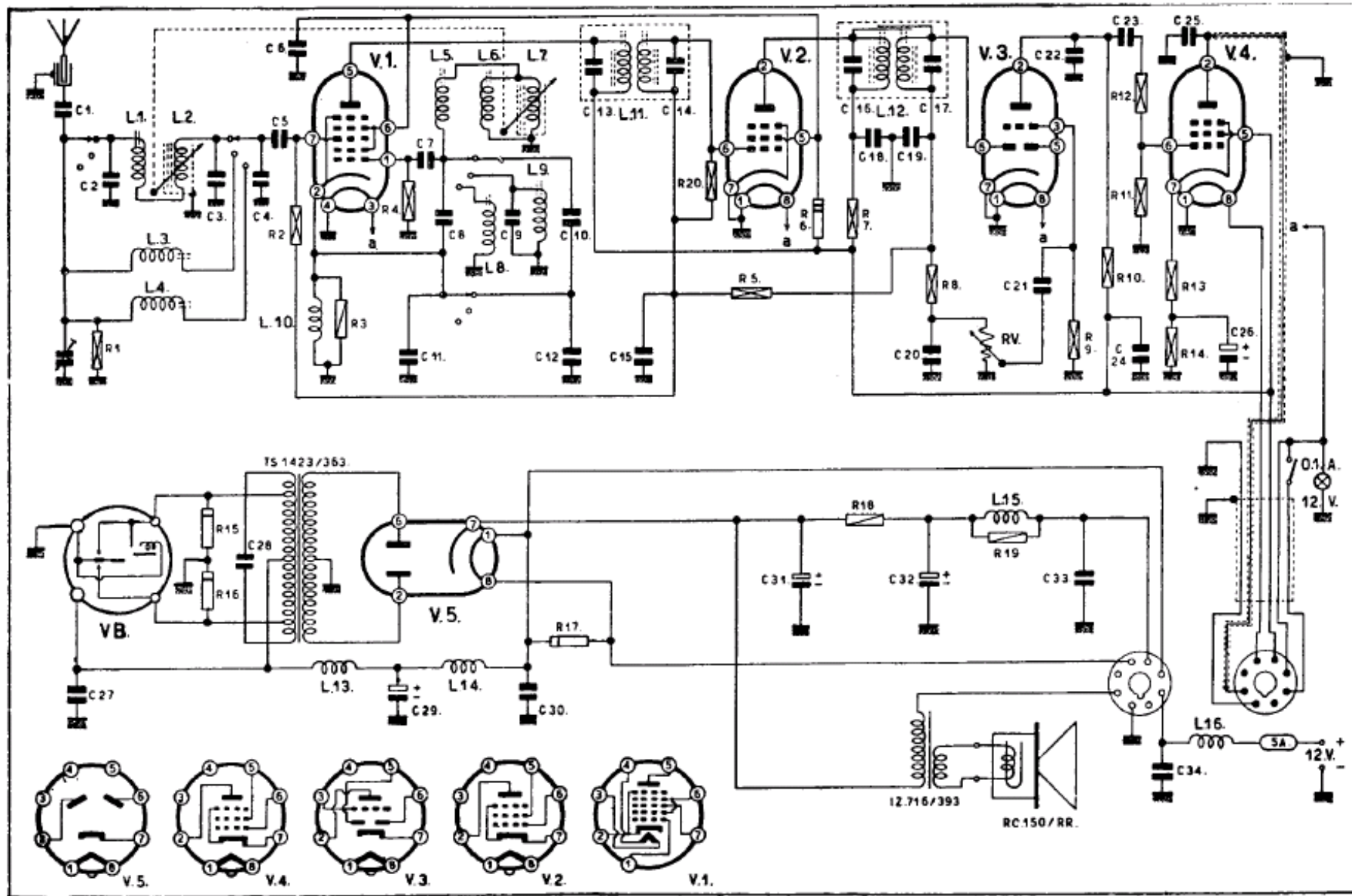
FIMI S.A. - PHONOLA - AUTORADIO mod. 5559. Onde medie e due onde corte. Media frequenza 470 kc/s.
